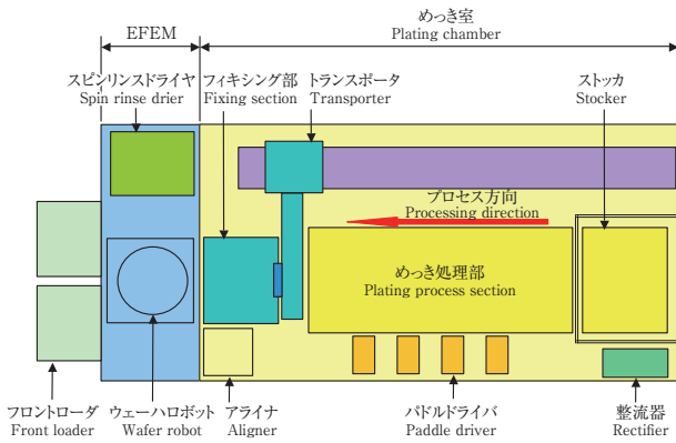
図1 装置構成 Fig. 1 System configuration
