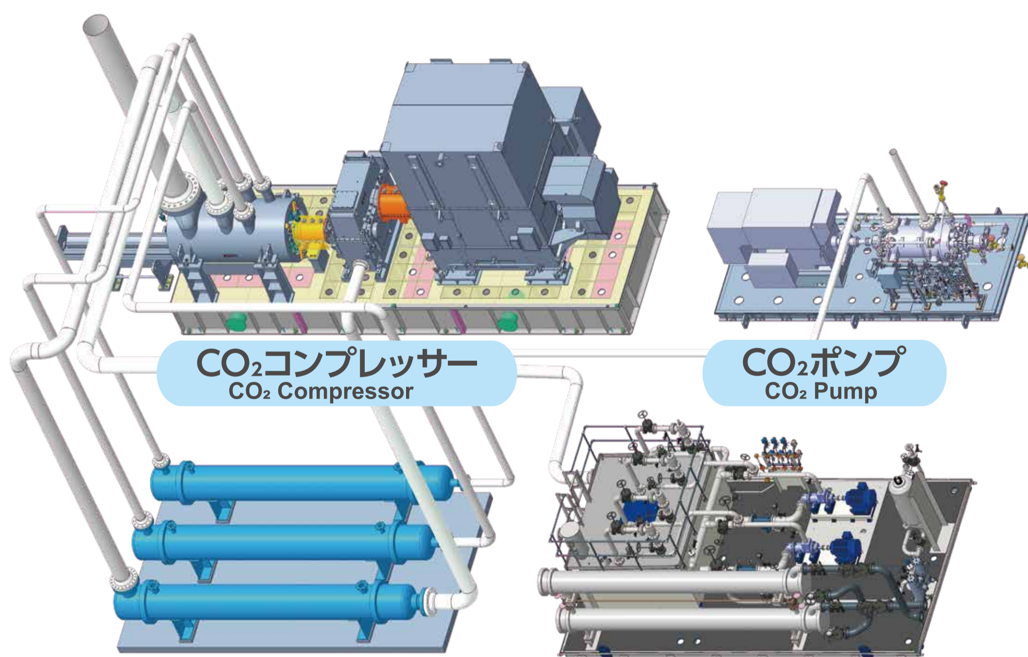
CO 2 Phase コンプレッサー&ポンプ ハイブリッドシステム CO 2 Phase Hybrid Compressor Pump Solution
